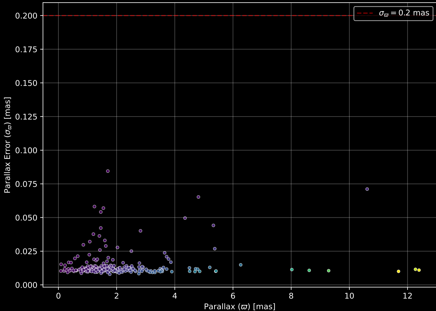
GALAH DR4 Field: [355] Parallax Quality (n= 287)
