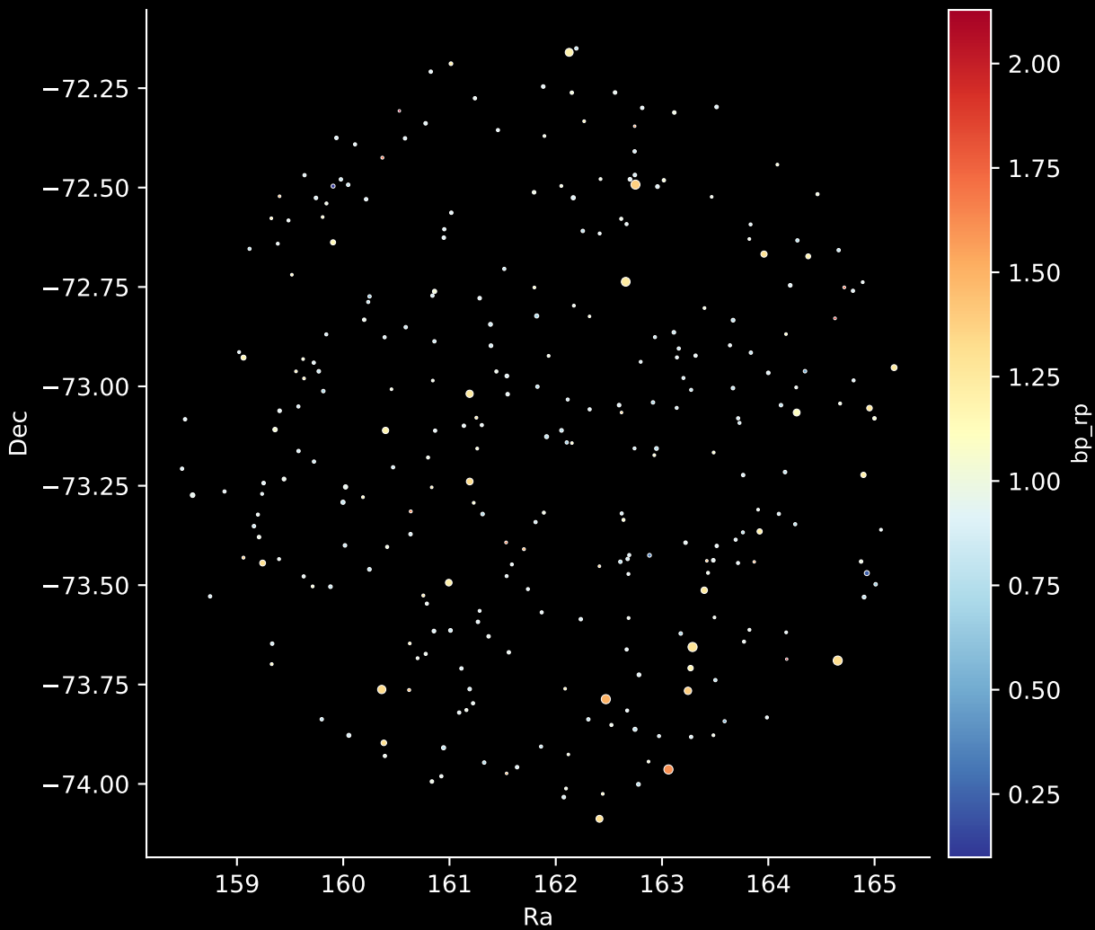
GALAH DR4 Field: [355] Stars: 287
