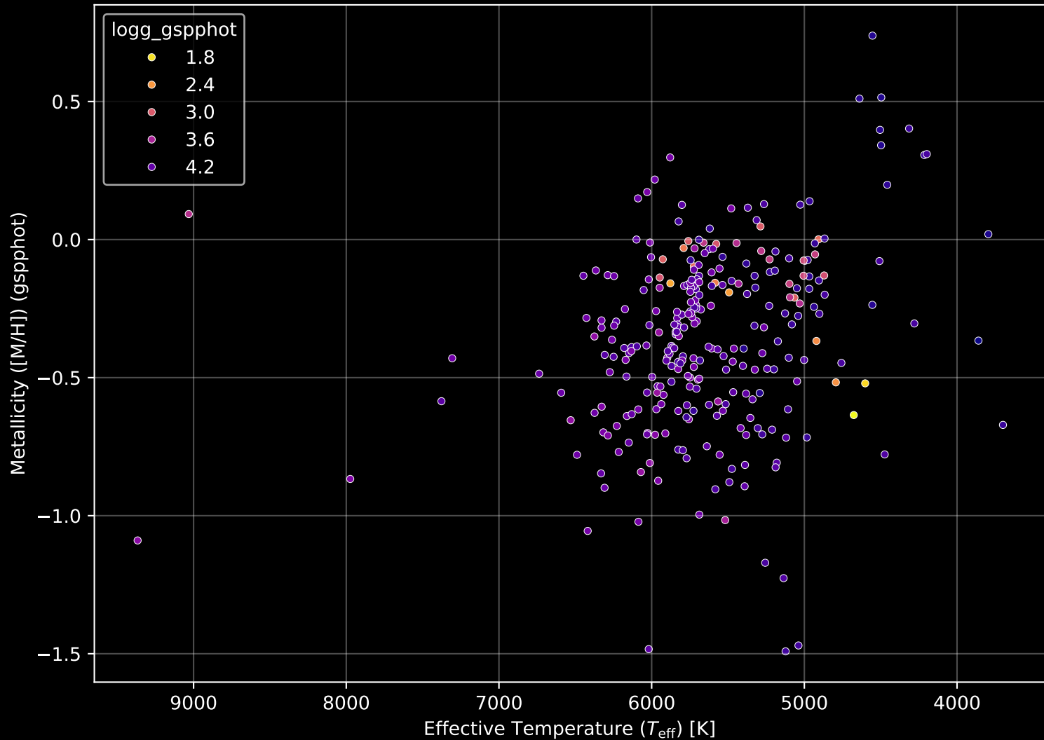
GALAH DR4 Field: [355] Stellar Population Parameters (n= 287)
