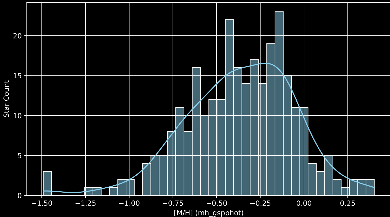
GALAH DR4 Field: [355] [M/H] (mh_gspphot) (n= 284)
